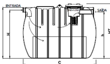
Fossa Séptica de 3000 litros
